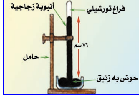
بارومتر تورشيلي
