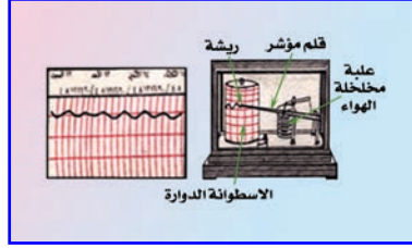
الباروجراف
