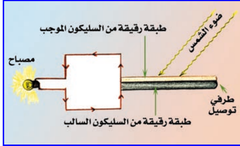
الخلية الشمسية
